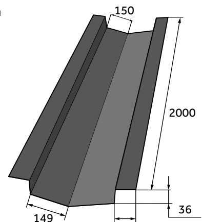
Figur 22: Kilrenne overbeslag 2000
