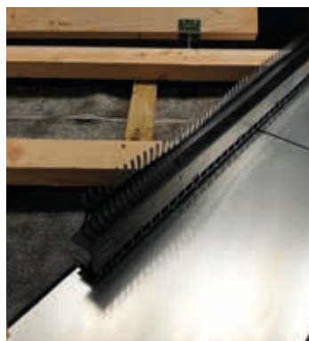
1 IcoVenti skotrendeelementer monteres fra kippen og ned mod tagfoden.
