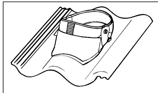
BRAMAC MAX - Průchozí taška DuroVent PLUS
