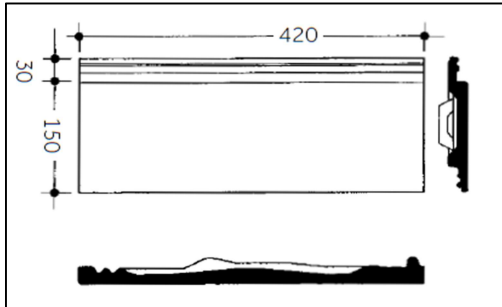
Technický výkres - střešní taška 1/2 TE STAR, TE PP
