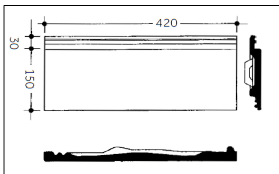
Technický výkres - Taška 1/2 TE STAR, TE
