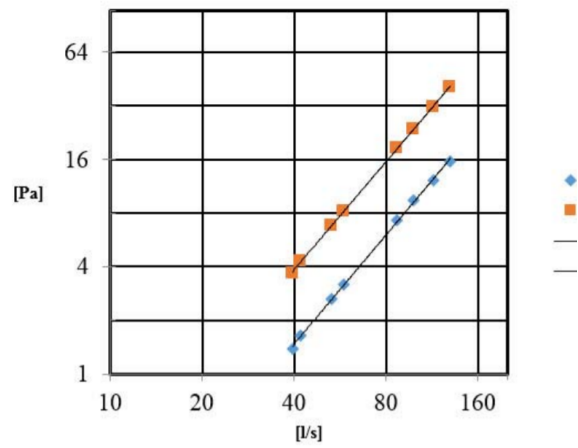
Tryckfallsdiagram vid 14° taklutning
