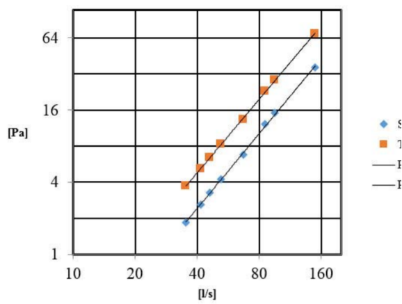
Tryckfallsdiagram vid 45° taklutning
