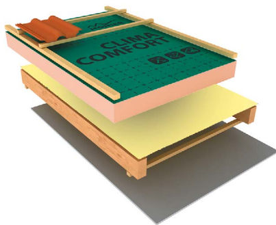
Enkel isolatie
