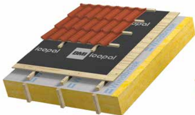
AeroDek Tradition Plus på bærende undertak, tekket med Icopal Ultra D underlagsbelegg
