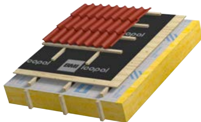
AeroDek ståltakplater på bærende undertak, tekket med Icopal asfalt underlagsbelegg og opplekting over vindspærresjiktet.
